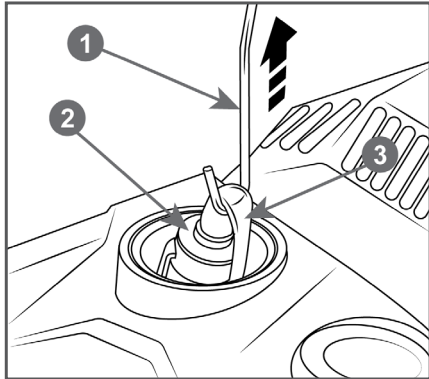
Рис. 22 Обслуживание топливного фильтра
