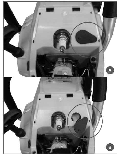
Рис. 10 Положение заслонки «зима-лето»
