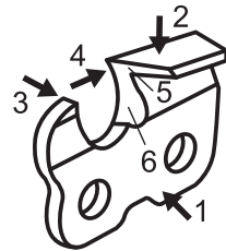
Рис. 31 Части режущего звена цепи
